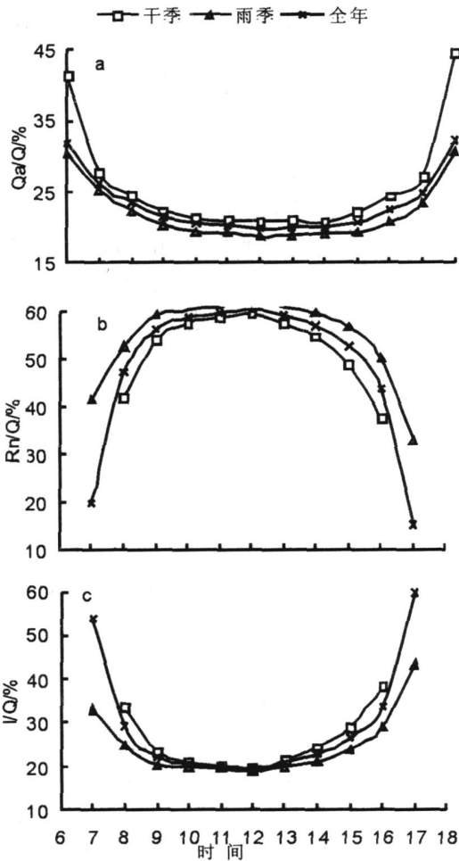
图 4 不同季节太阳辐射各分量 占总辐射分配率日的变化
