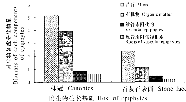
图 2 石林喀斯特森林群落中林木与岩石上附生物生物量的比较
