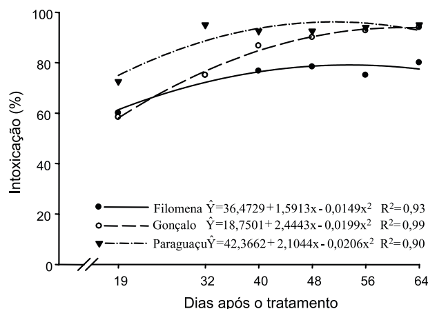
Figura 3 - Intoxicação de genótipos de pinhão-mansó pelo herbicida isoxaflutole. Viçosa-MG, 2009.
