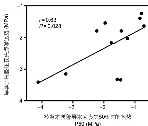
图3 西双版纳热带岩溶森林植物的枝条导水率丧失50%时的水势(P50)与叶片旱季膨压丧失点水势之间的相关关系
