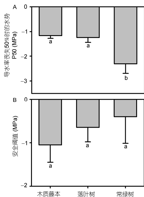
图2 热带岩溶落叶(6种)、常绿树木(6种)和木质藤本(13种)木质部导水率丧失50%的水势(P50)和安全边界(植物最低水势-P50)比较
