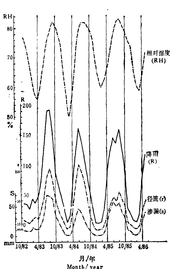
图 2(a) 降雨、径流、渗漏及相对湿度曲线
