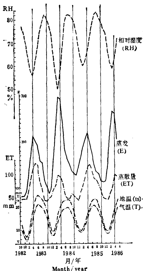
图 2(b) 蒸发、蒸散、地温、气温及相对湿度
