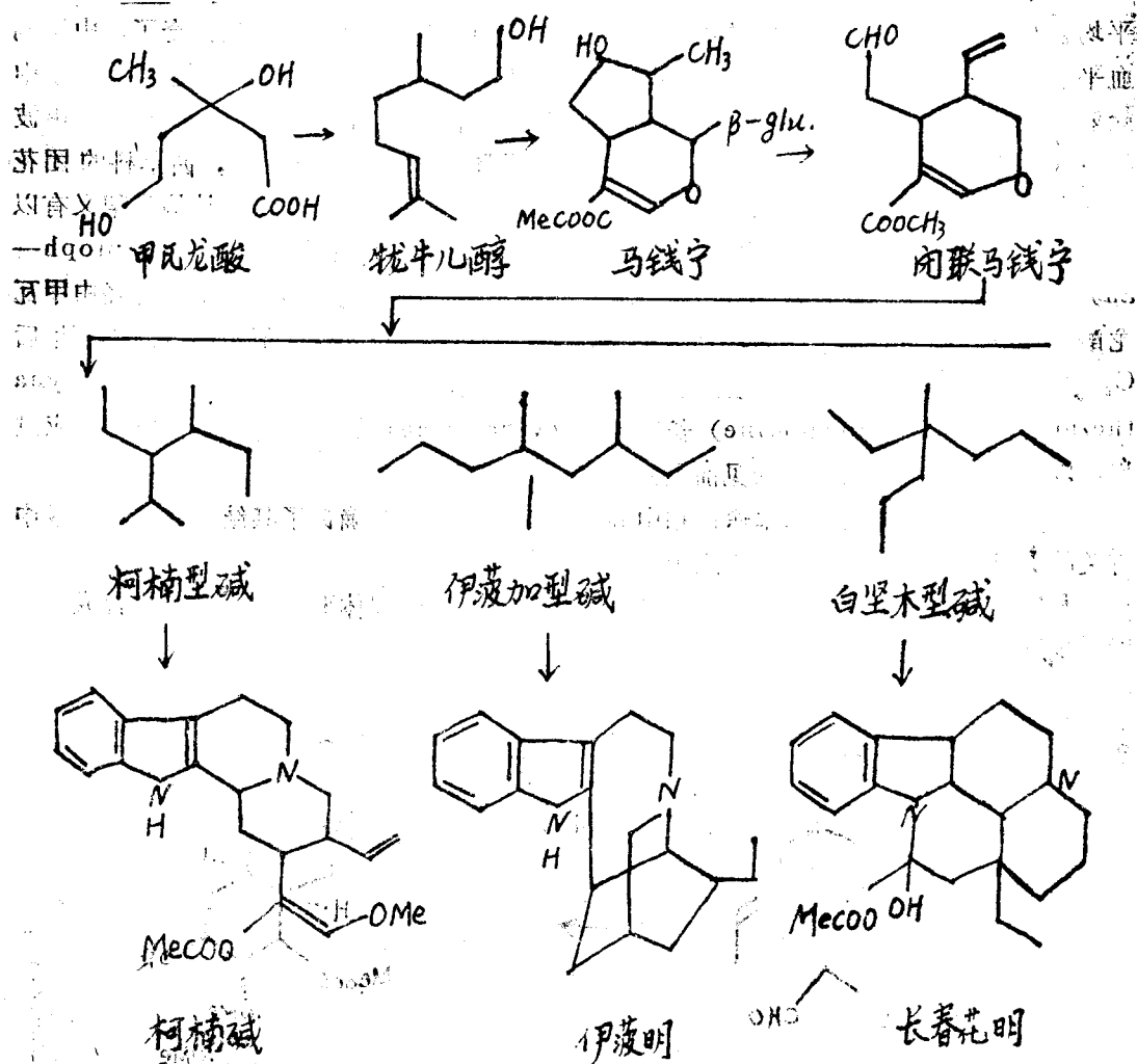
图 1. 柯楠碱, 伊波明, 长春花明生物碱的次级代谢途径
