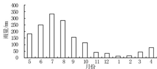
图 2 1992~2006 期间降雨年内分配情况(水文年)
