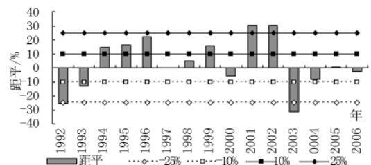
图 1 勐仑年降雨量距平百分比 相对于 1959~1998 年平均值
