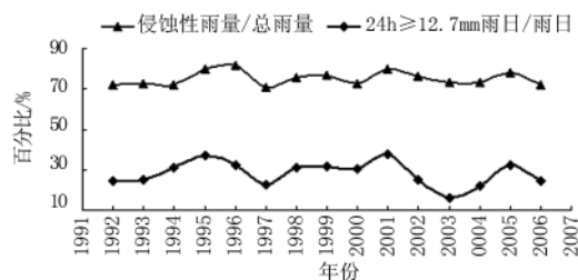
图 3 侵蚀性雨量/总雨量、 24 h \geq 12.7 mm 雨日/雨日的百分比年变化
