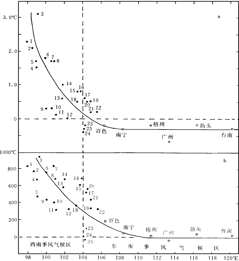
图3 中国南方北回归线附近的冠-气温差 \Delta T 分布
