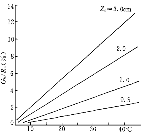
图 1 不同 Z_b 值条件的 G_b/R_n (%) 与中国南方温度年较差( \Delta T_a ) 的关系
