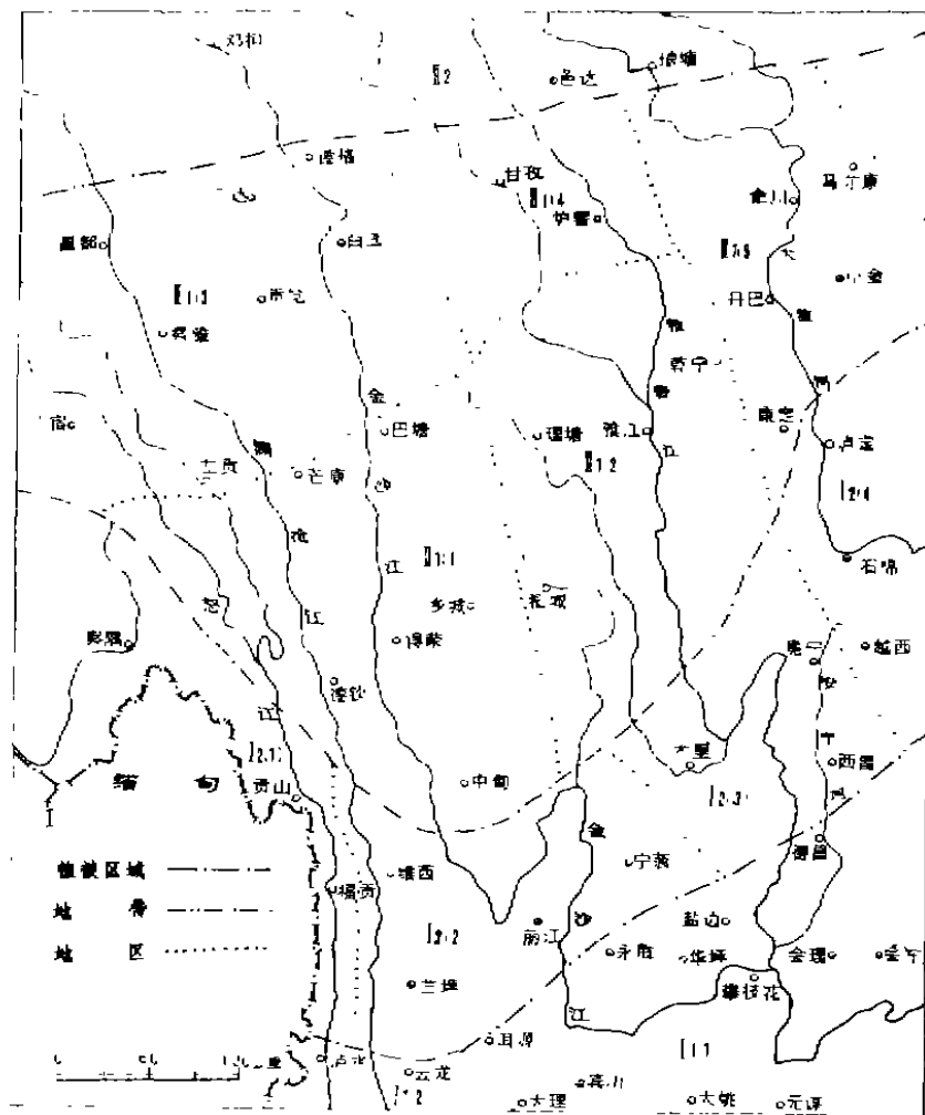
附图 横断山区植被分区图
