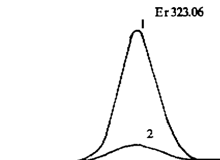
图 1 Sm 对 Er 的干扰图
