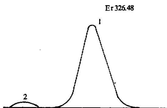
图 2 Er 无干扰图
