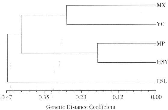
图1 流苏石斛居群基于 Nei's 遗传距离的UPGMA 聚类图
