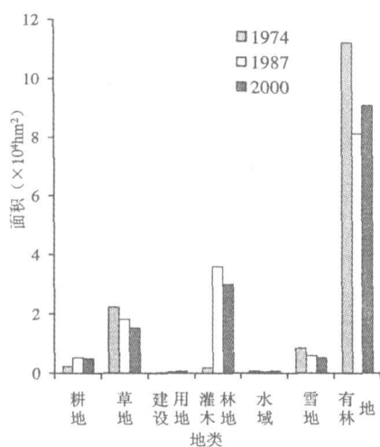
图 3 建塘镇 (1974~ 2000)土地利用 /覆盖的变化
