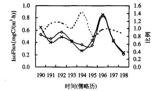
图 4 异戊二烯排放通量的观测值和计算值以及二者之比
