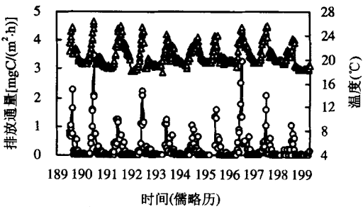
图 1 异戊二烯排放通量和气温的变化曲线 Fig.1 The variation curves of isoprene emission flux and air temperature —○— 排放通量 —△— 温度
