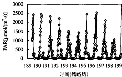
图 2 光合有效辐射的变化曲线 Fig.2 The variation curve of PAR
