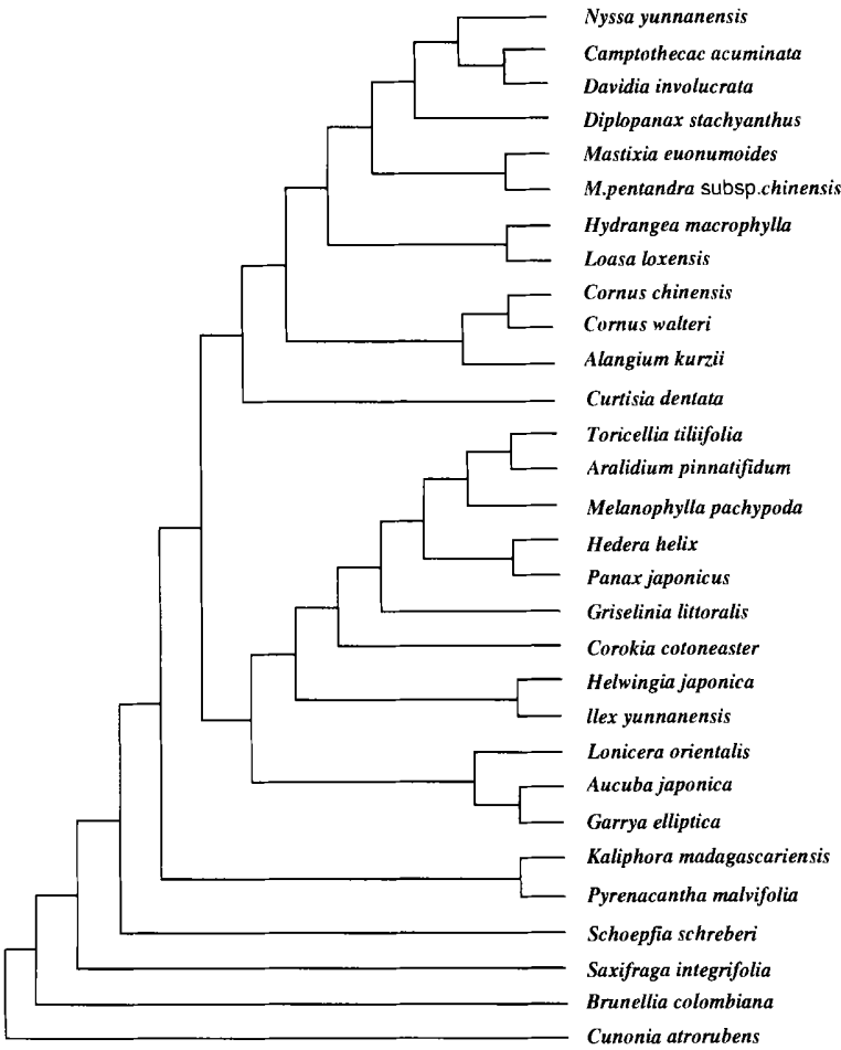
图 1 PAUP 分析 rbcL 序列所得的 24 棵最简约分支树图 (分支图步长= 865 步, CI= 0.5283, RI= 0.4756) 之一。 Cunonia atrorubens 、 Brunellia colombiana 和 Saxifraga integrifolia 为外类群。
