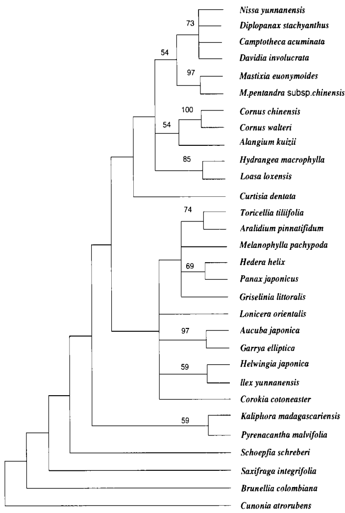
图 2 24 棵最简约树的严格一致树。靴带分析值位于分支的上方
