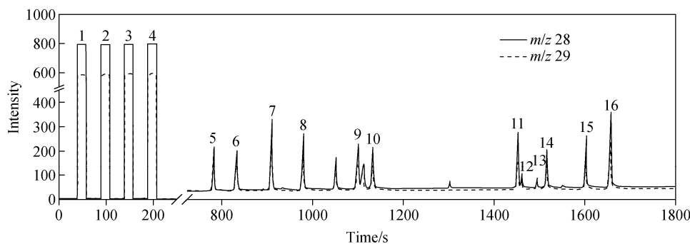
注: 1~4 为 \text{N}_2 参比峰, 5~16 分别为丙氨酸、甘氨酸、 \alpha -氨基丁酸、缬氨酸、亮氨酸、异亮氨酸、天冬氨酸、苏氨酸、丝氨酸、蛋氨酸、谷氨酸和苯丙氨酸的 \text{N}_2 样品峰
