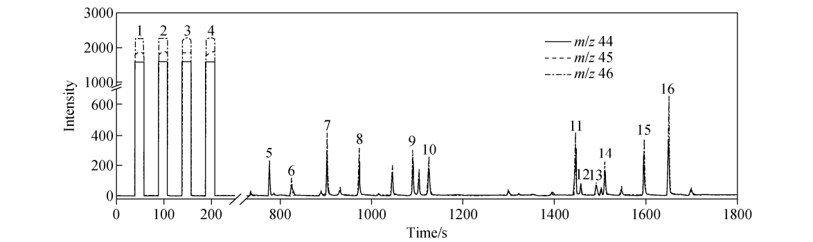
注:1~4为 \text{CO}_2 参比峰,5~16分别为丙氨酸、甘氨酸、 \alpha -氨基丁酸、缬氨酸、亮氨酸、异亮氨酸、天冬氨酸、苏氨酸、丝氨酸、蛋氨酸、谷氨酸和苯丙氨酸的 \text{CO}_2 样品峰 图3 GC-C-IRMS测定混合体系中特定氨基酸 \delta^{13}\text{C} 的色谱图 Fig. 3 Chromatogram of specific amino acid \delta^{13}\text{C} by GC-C-IRMS
