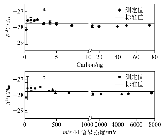
图 1 GC-C-IRMS 测定咖啡因 \delta^{13}\text{C} 的进样量(a)和信号强度(b)响应特征
