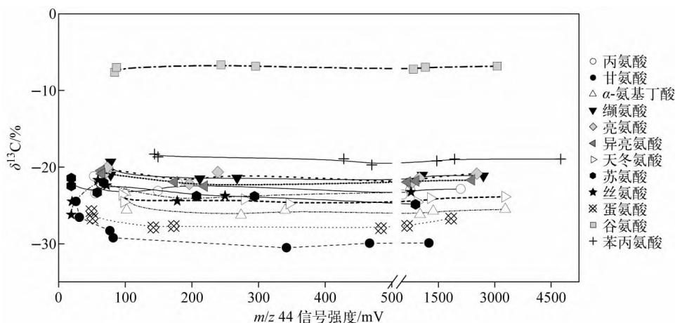
图4 GC-C-IRMS 测定混合体系中特定氨基酸 \delta^{13}\text{C} 的信号强度依赖性特征
