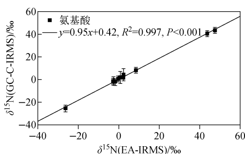
图6 GC-C-IRMS与EA-IRMS 测定氨基酸 \delta^{15}\text{N} 的对比
