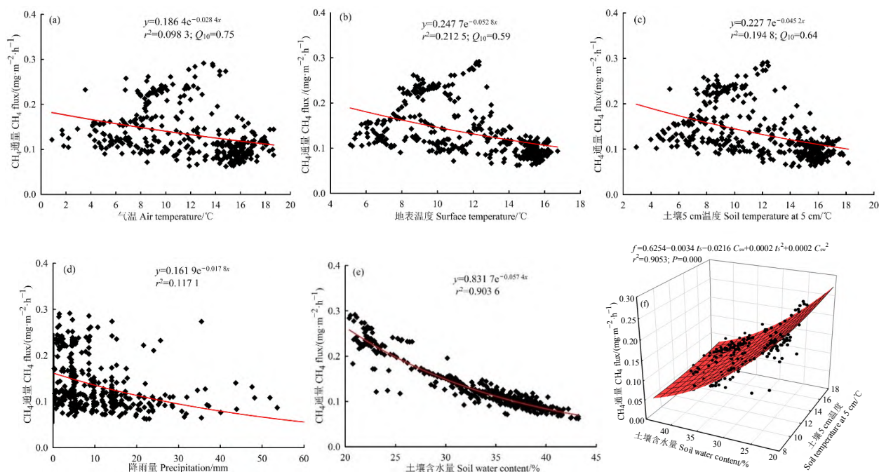
图3 温度、土壤含水量与土壤 \text{CH}_4 通量的指数回归及其双因子交互作用关系
