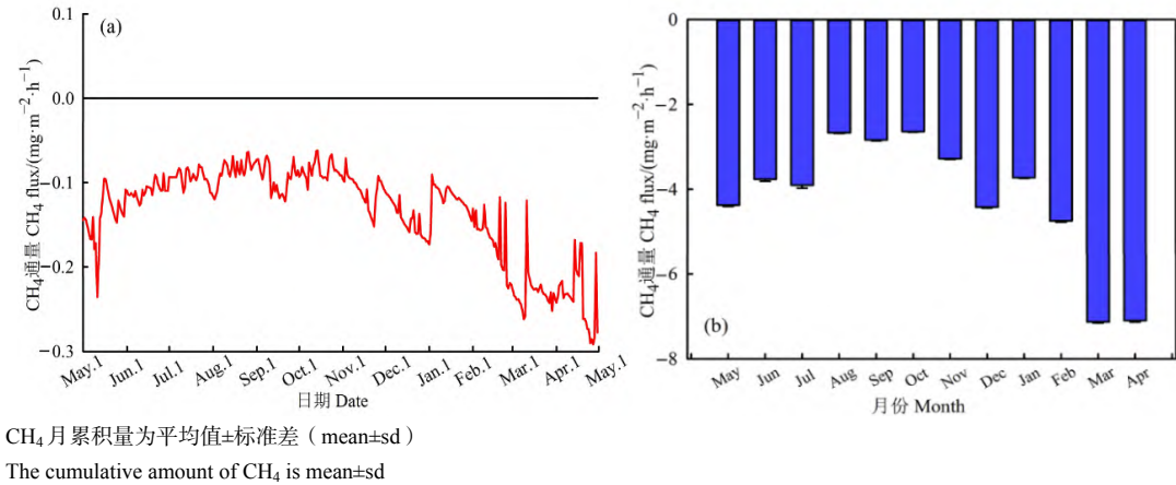
图 2 土壤 CH 4 日动态 (a) 和月累积通量 (b)
