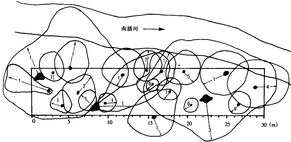
图 2 东京枫杨群落水平投影图 Fig. 2 The projection map of Pterocarya tonkinensis community
