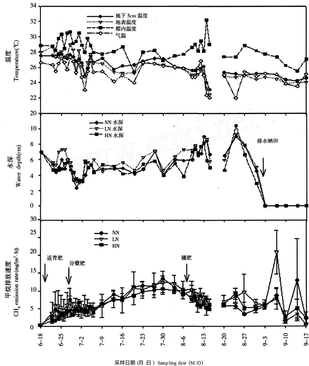
图 1 稻田温度、水深及 CH 4 排放通量的季节变化
